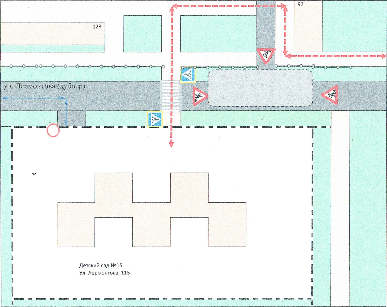
План-схема пути движения транспортных средств и воспитанников при проведении дорожно-строительных работ вблизи образовательного учреждения
